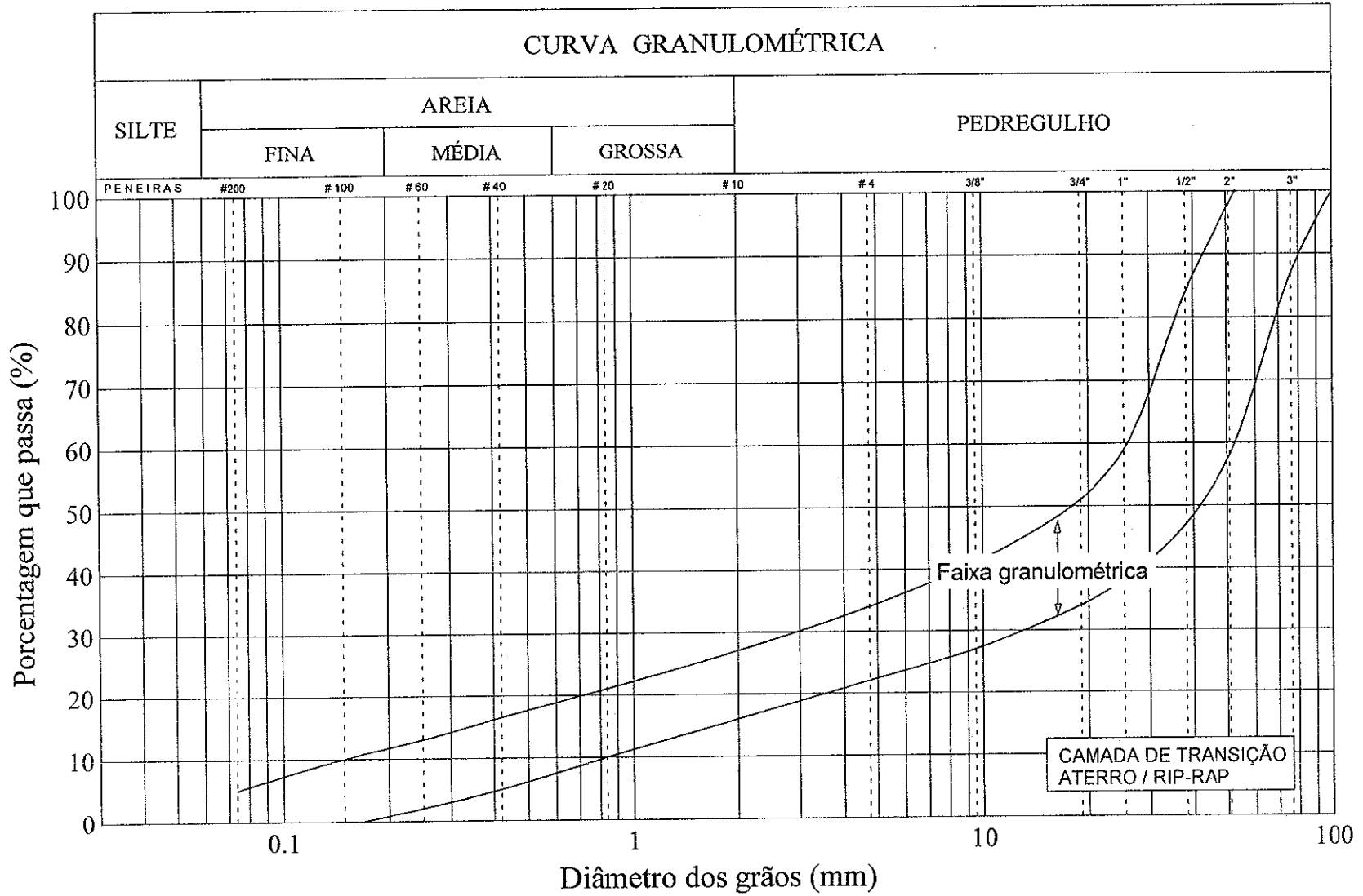
Figura 7.2 - Composição granulométrica da camada de transição entre o aterro compactado e o rip-rap
