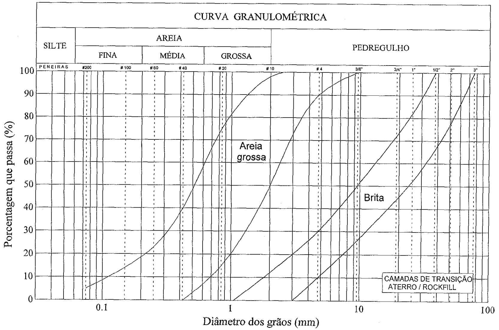
Figura 7.1 - Composição granulométrica das camadas de transição entre o aterro compactado e o rockfill
