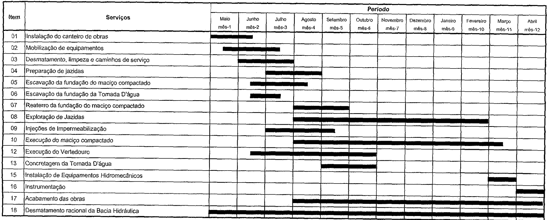
FIGURA 2.1 CRONOGRAMA FÍSICO - BARRAGEM FAÉ
